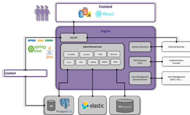
Εικόνα 15: Προτεινόμενη Αρχιτεκτονική Λύση
